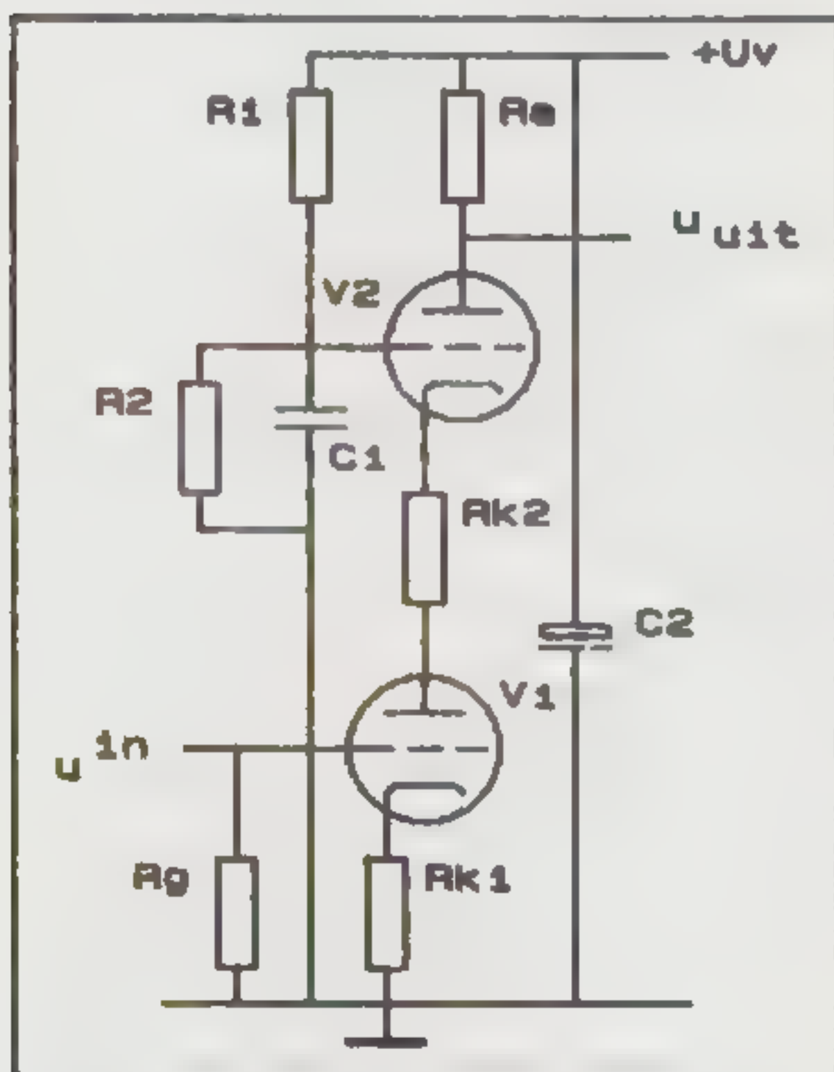
Figuur 17 Cascode schakeling
